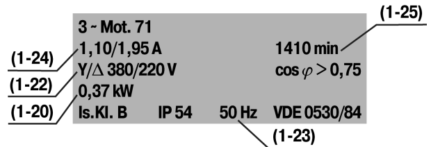
Шильдик двигателя (пример). В скобках указаны номера параметров для ввода в ПЧВ
